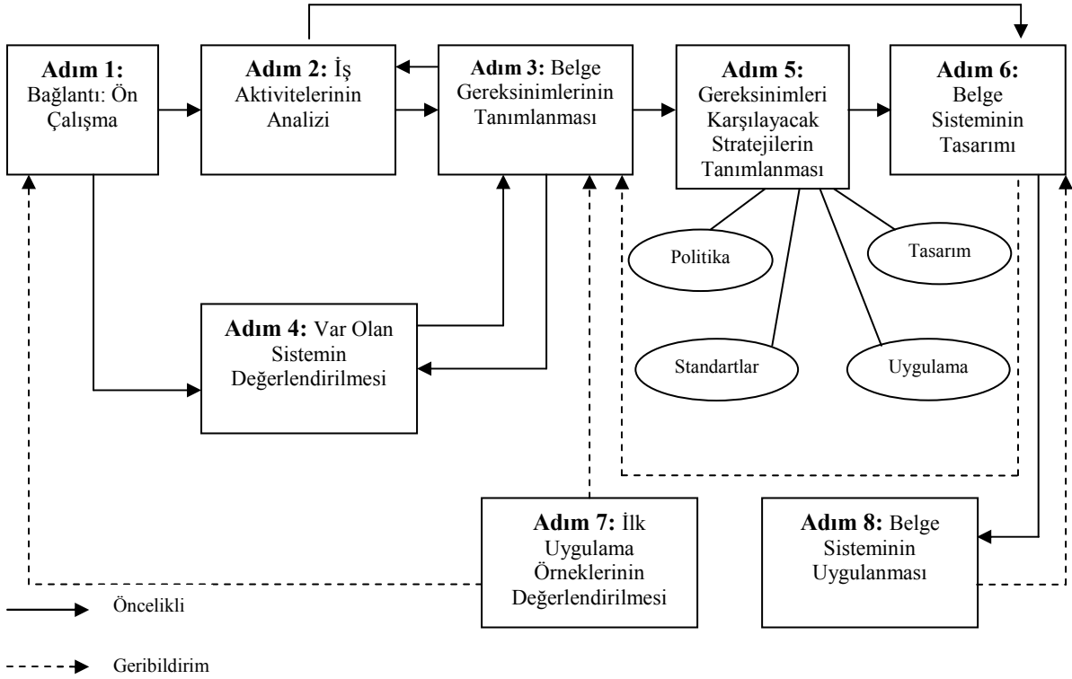
Şekil 1. Belge Yönetim Sistemlerinin Tasarımı ve Uygulanması (Brumm, 2005:32)
